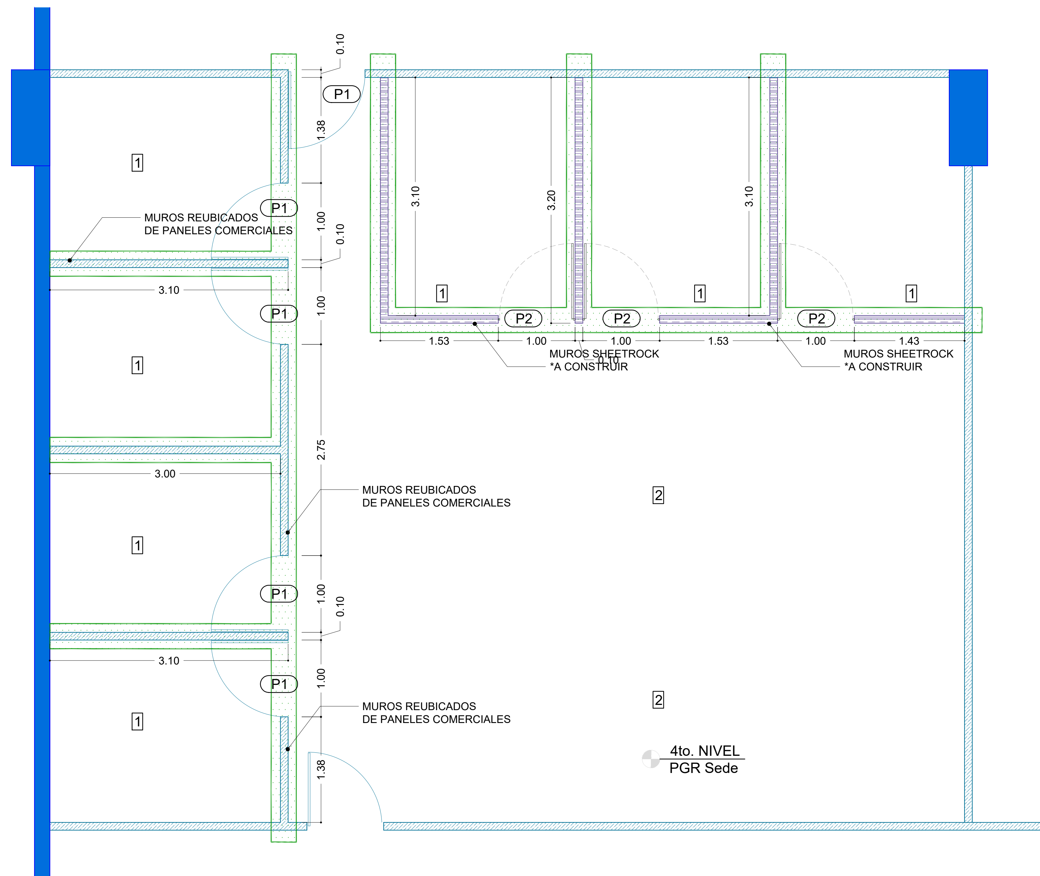
PLANTA DE TRABAJO - A CONSTRUIR DEPTO. DICTÁMENES - PGR SEDE
