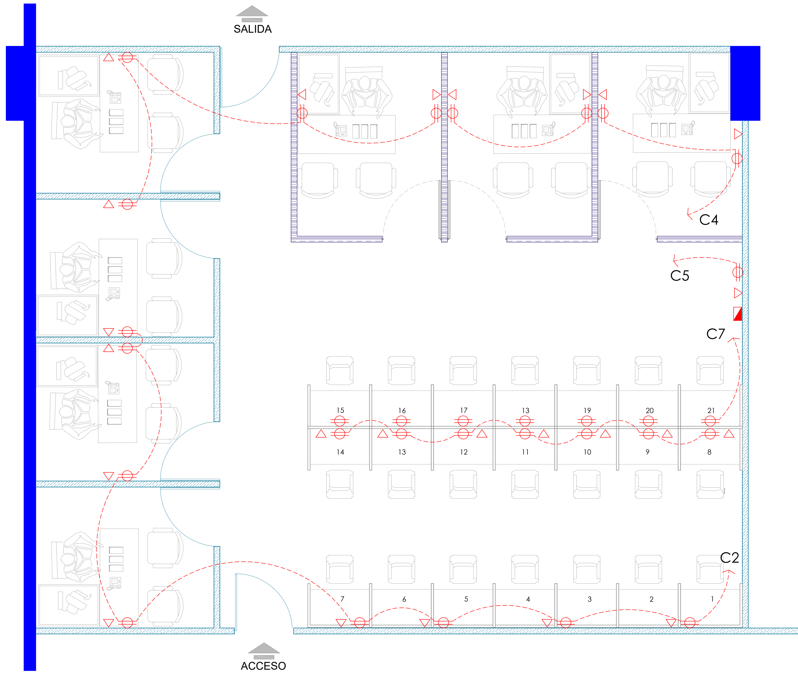
PLANTA DE DISTRIBUCIÓN TOMACORRIENTES DICTÁMENES- PGR SEDE
