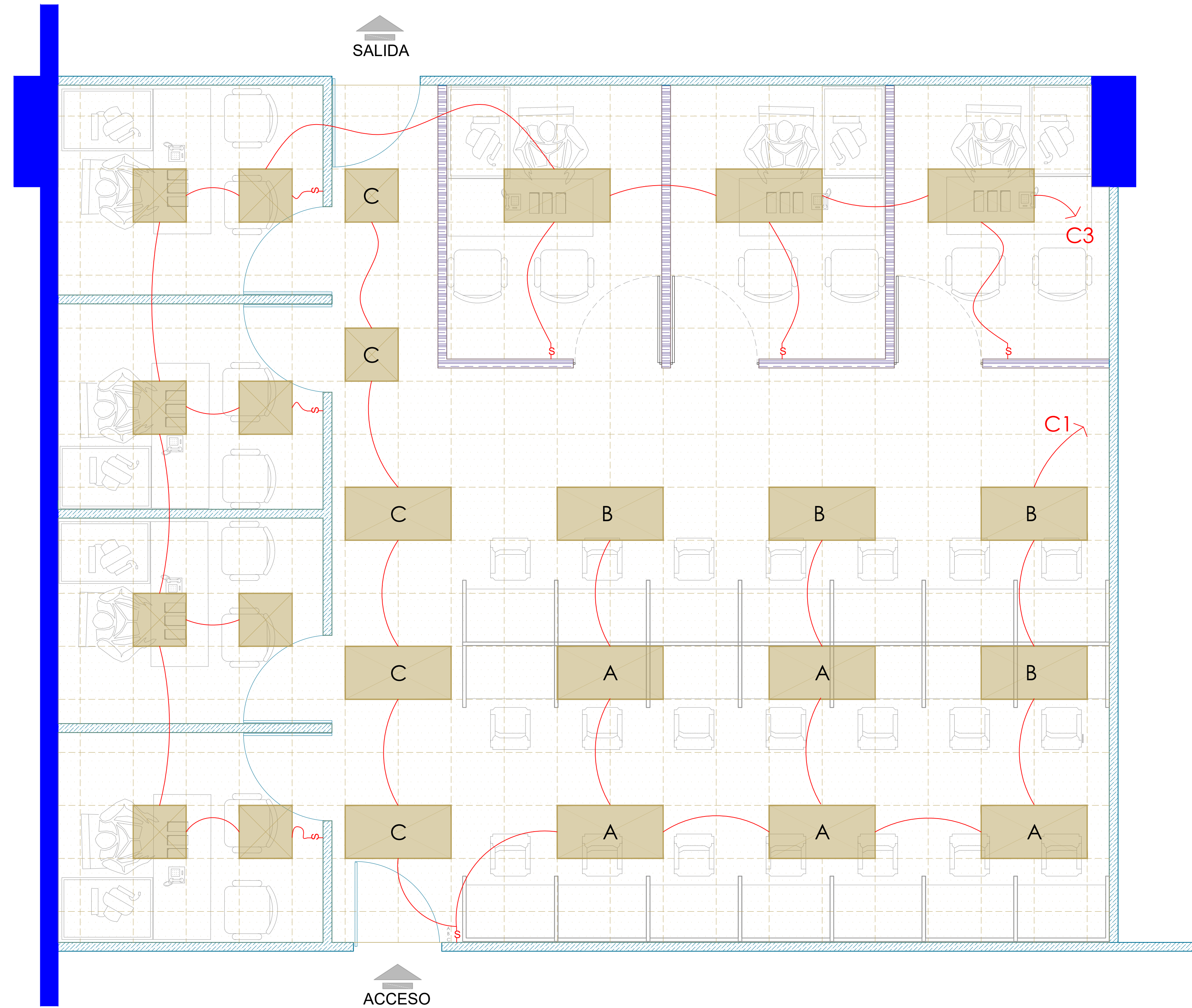
PLANTA DE DISTRIBUCIÓN DE LUMINARIAS DICTÁMENES- PGR SEDE
