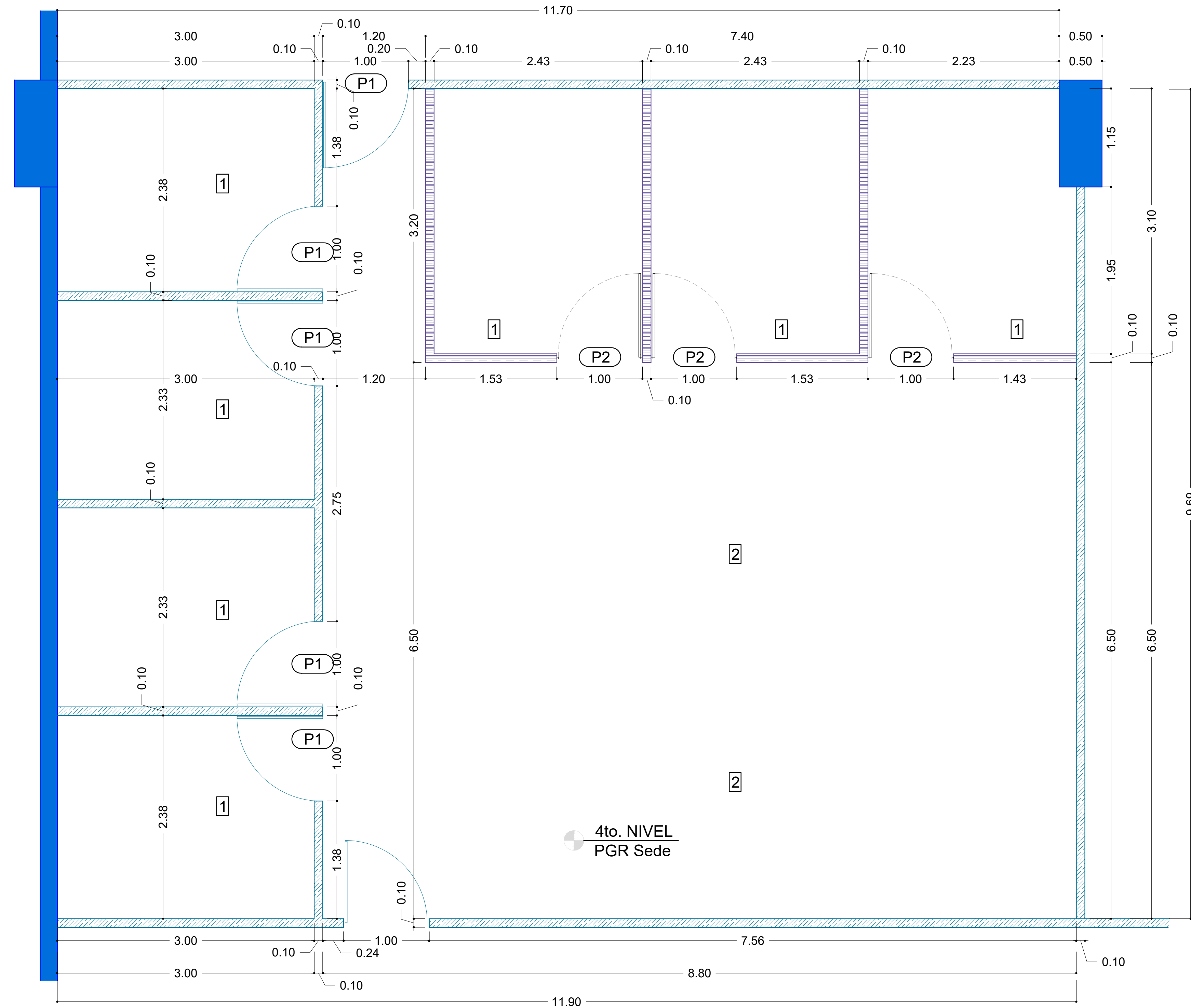
PLANTA DIMENSIONADA DEPTO. DICTÁMENES - PGR SEDE
