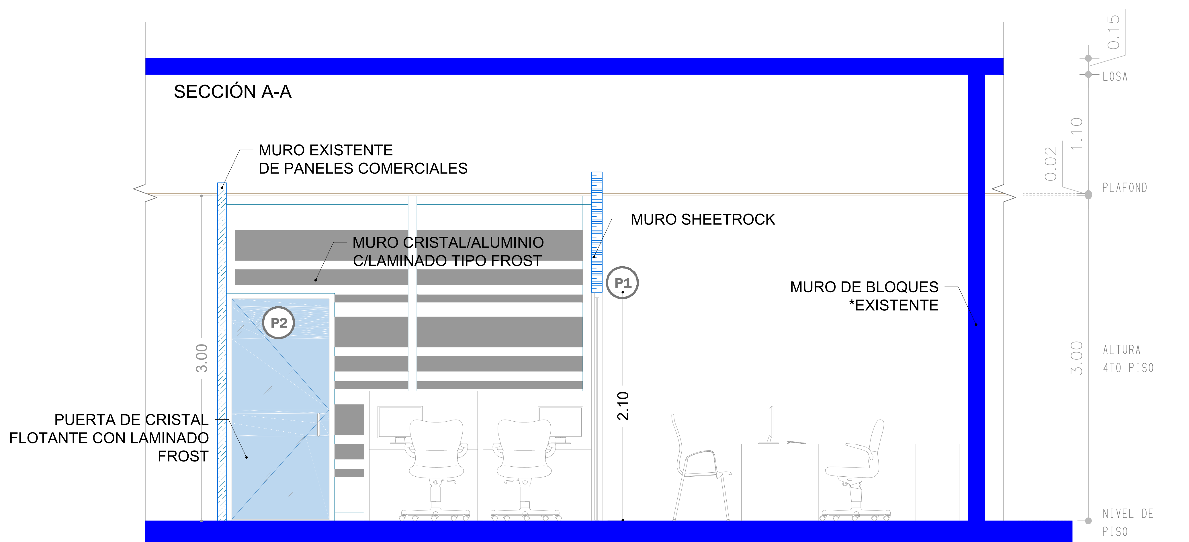
SECCIÓN A-A' ESC 1:20
