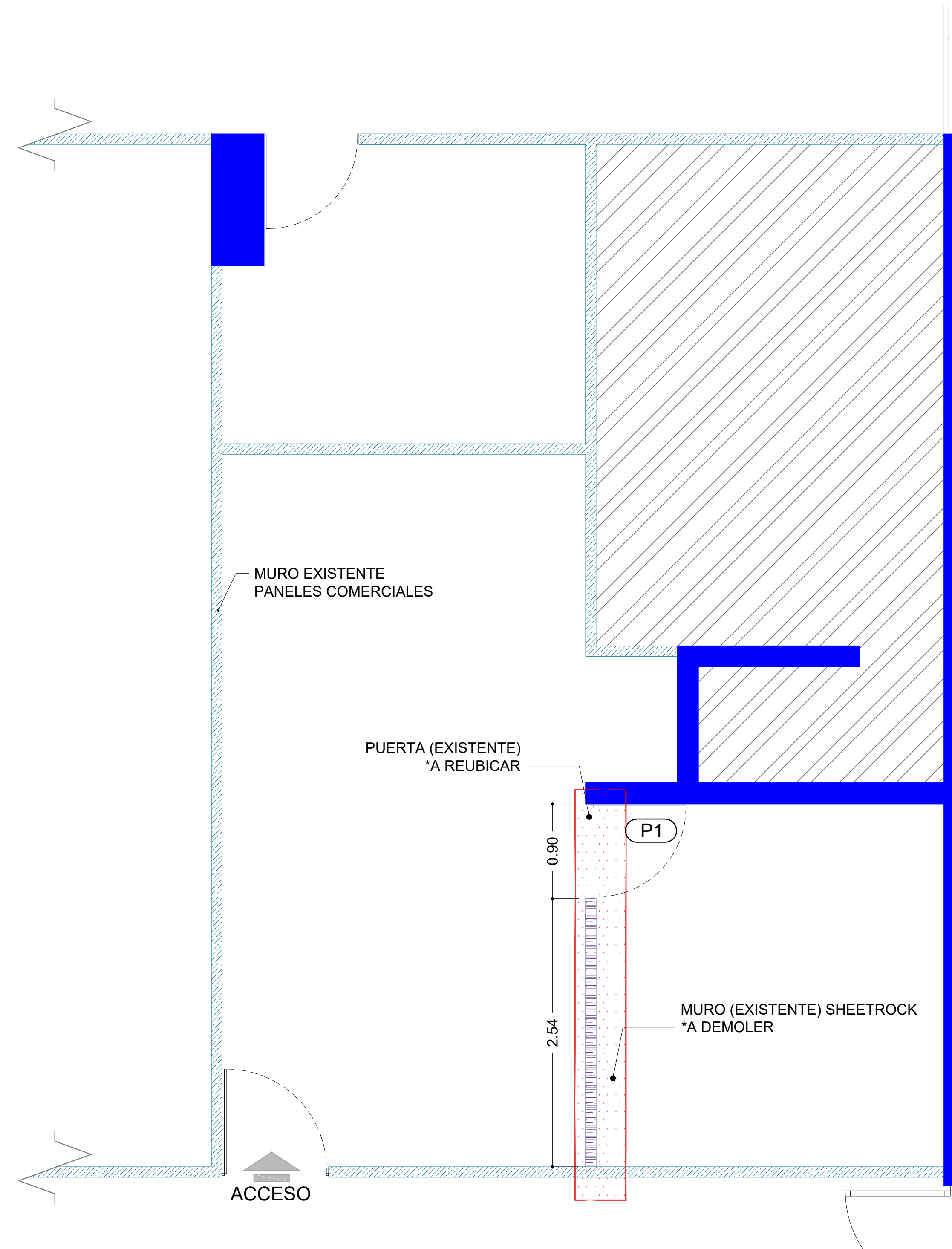
PLANTA DE TRABAJO - A DEMOLER DCI LOTE 1- PGR SEDE
