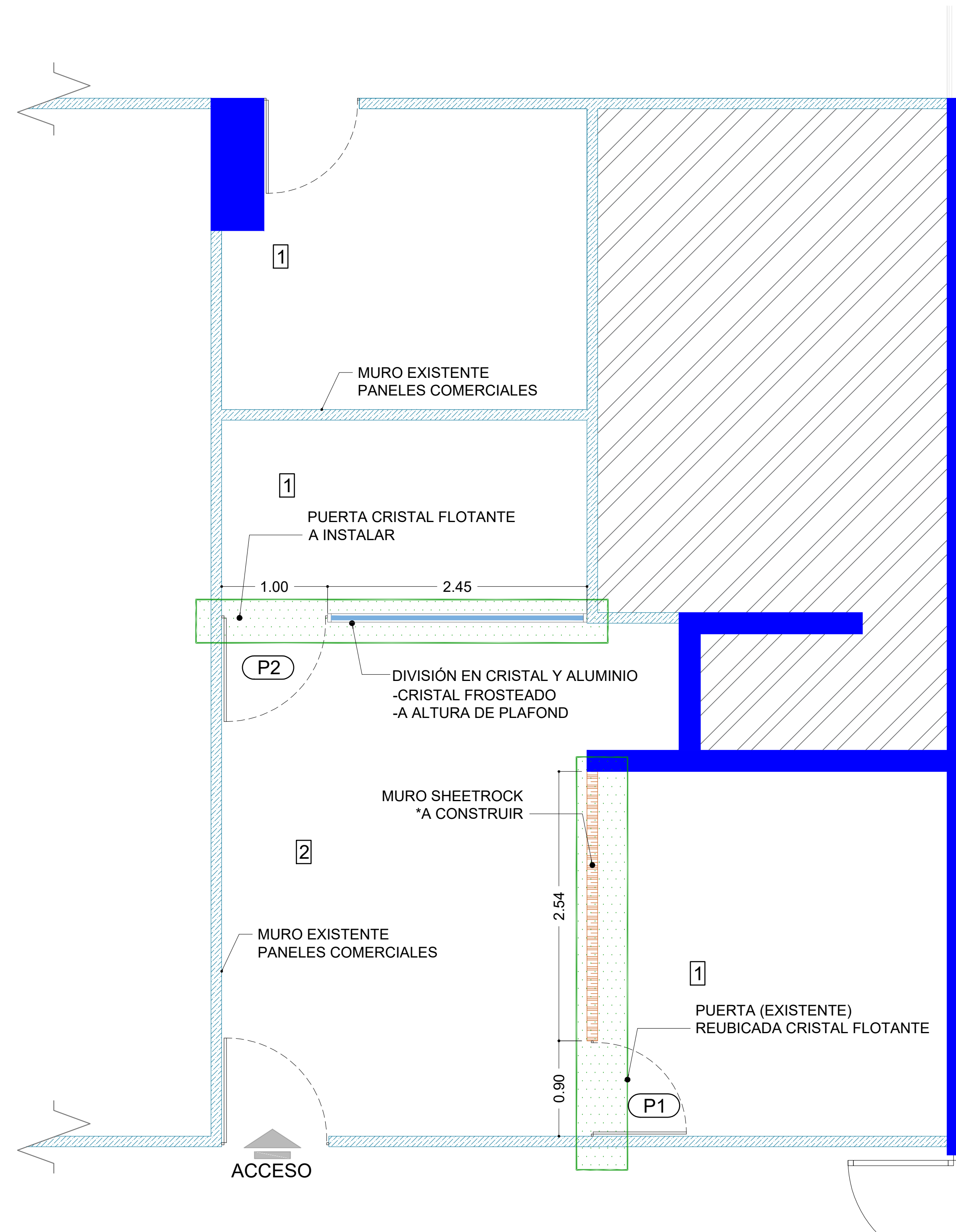
PLANTA DE TRABAJO - A CONSTRUIR DCI LOTE 1- PGR SEDE
