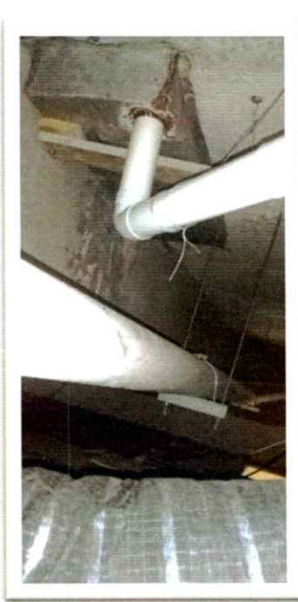
BANDEJAS DE DRENAJE PLUVIAL CORROIDAS
