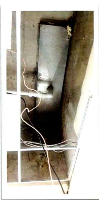
BANDEJAS DE DRENAJE PLUVIAL CORROIDAS
