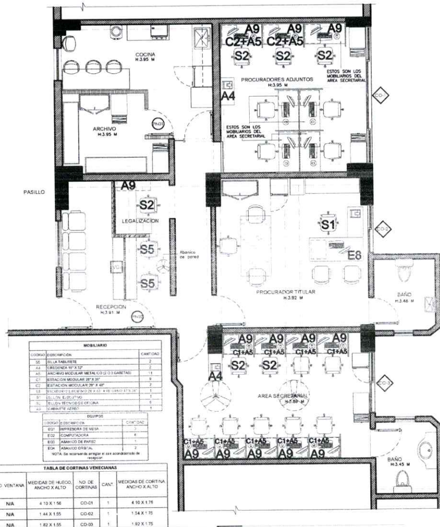
PLANTA: PLANO DE MOBILIARIOS ESCALA: 1/90
