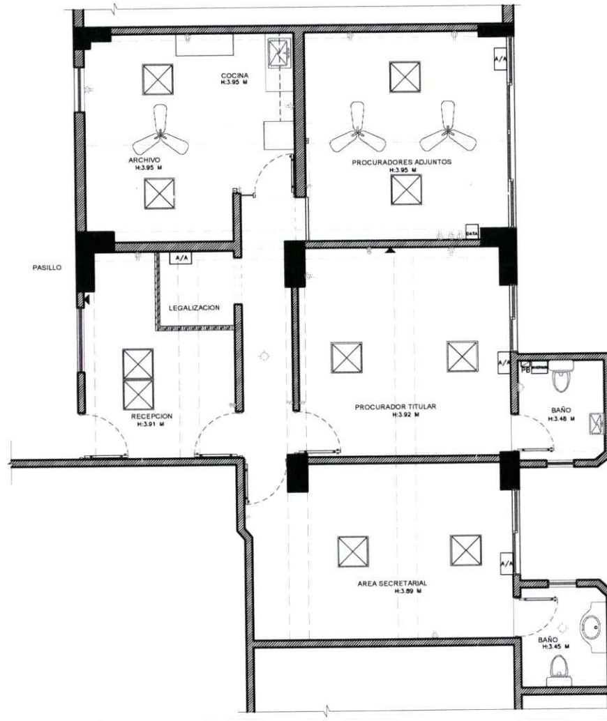
PLANTA: LEVANTAMIENTO ELECTRICO ESCALA: 1/90
