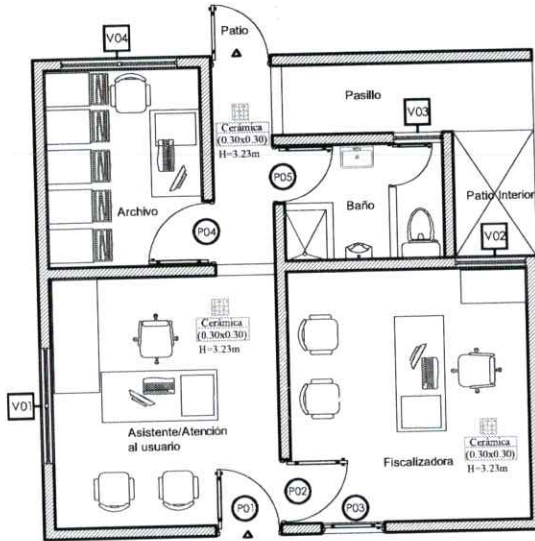
PLANTA: ARQUITECTONICA JUZGADO DE PAZ NIGUA (AREA MF) ESCALA: 1/100
