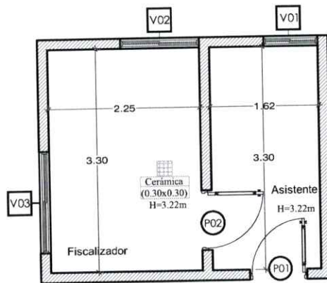
PLANTA: DIMENSIONADA JUZGADO DE PAZ BAJOS DE HAINA ESCALA: 1/75
