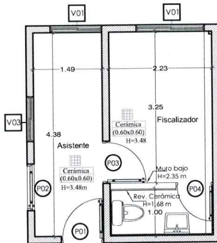
PLANTA: DIMENSIONADA SEDE POLICIAL BAJOS DE HAINA ESCALA: 1/75
