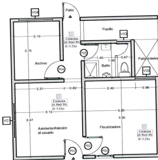
PLANTA: DIMENSIONADA JUZGADO DE PAZ NIGUA (AREA MF) ESCALA: 1/100
