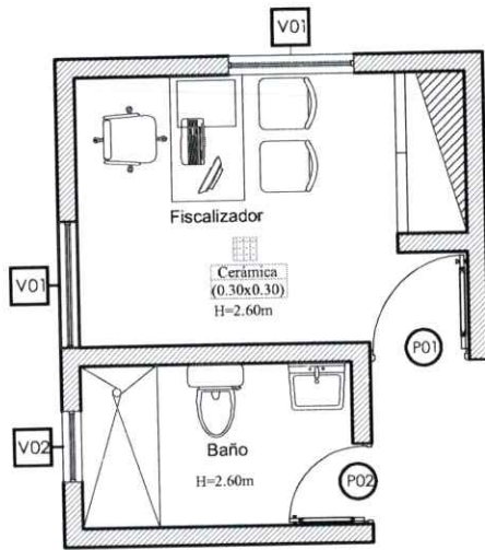
PLANTA: ARQUITECTONICA JUZGADO DE PAZ PALENQUE (AREA MP) ESCALA: 1/75
