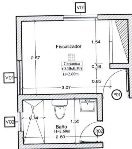
PLANTA: DIMENSIONADA JUZGADO DE PAZ PALENQUE (AREA MP) ESCALA: 1/75
