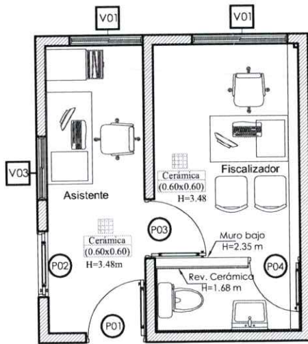
PLANTA: ARQUITECTONICA SEDE POLICIAL BAJOS DE HAINA ESCALA: 1/75
