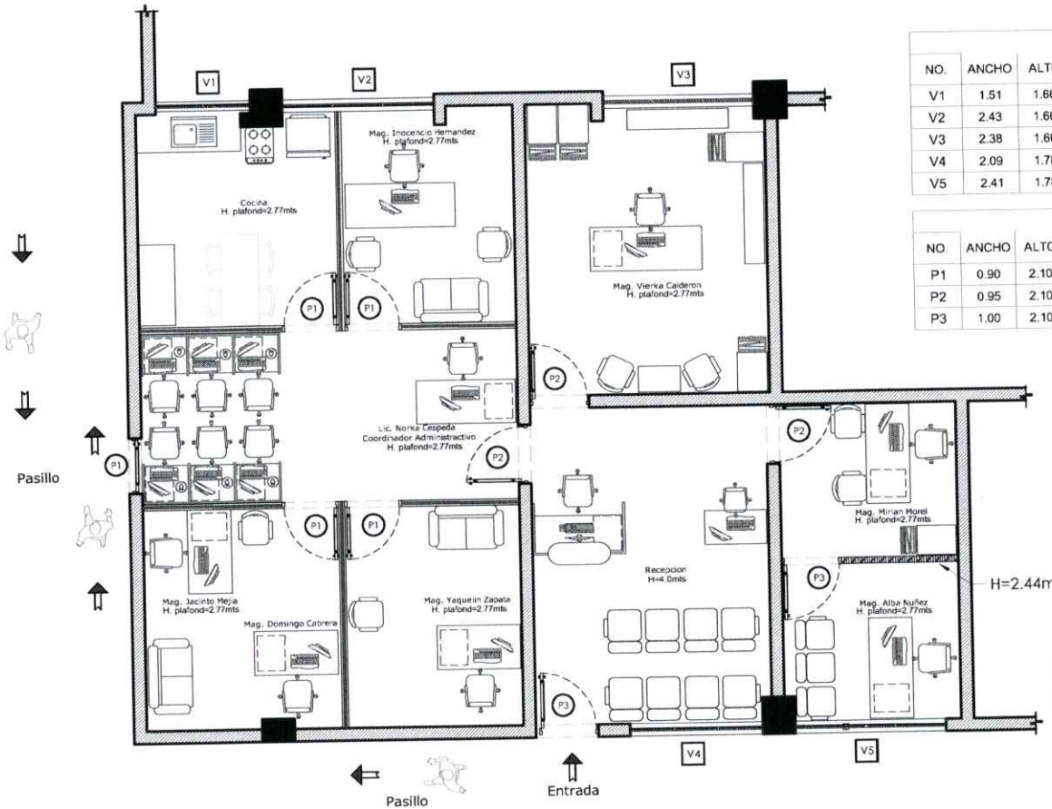
PLANTA: ARQUITECTONICA EXISTENTE ESC: 1:100 1ER NIVEL
