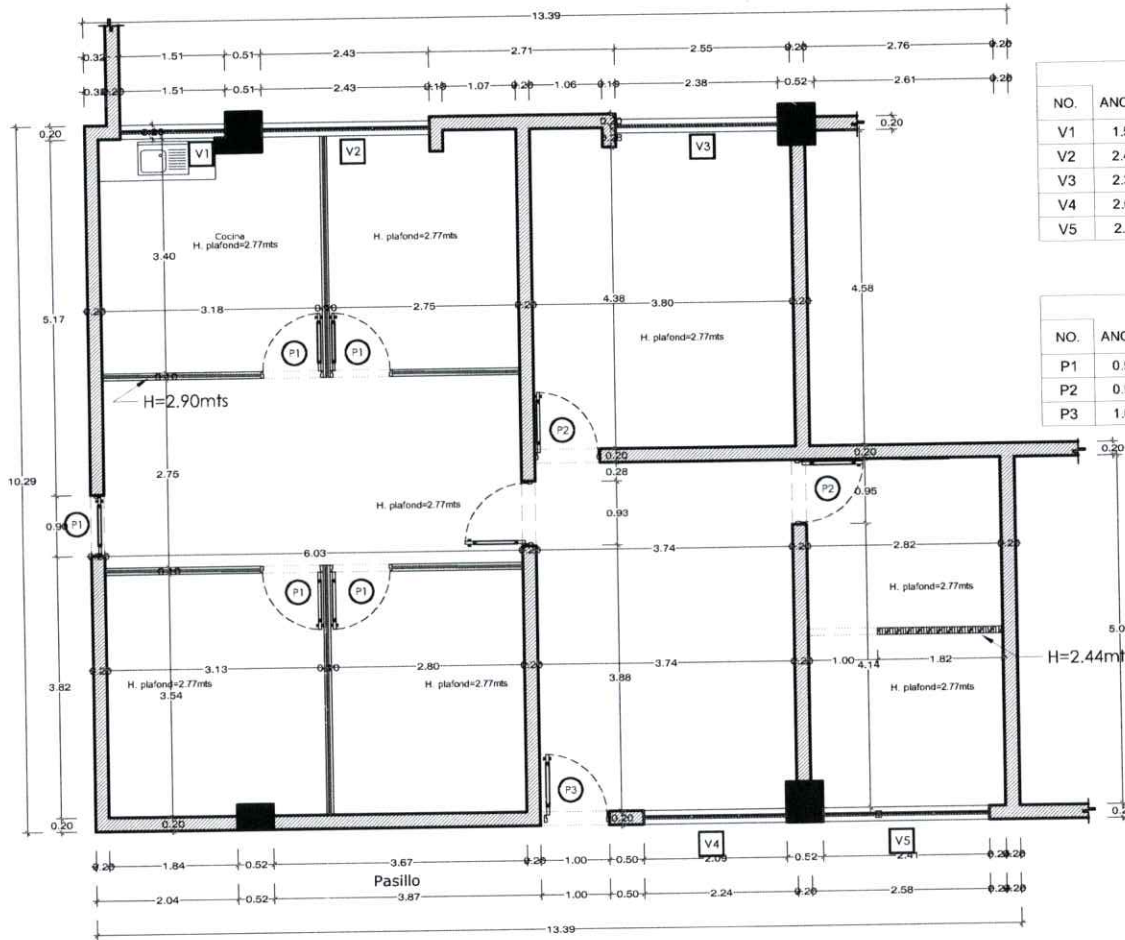
PLANTA: DIMENSIONADA EXISTENTE ESC: 1:100 1ER NIVEL
