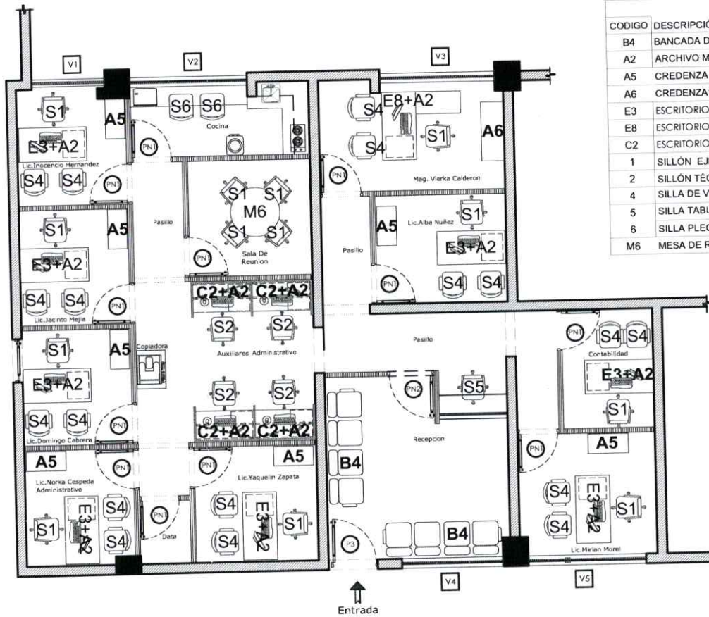
PLANTA: MOBILIARIOS ESC: 1:100 1ER NIVEL
