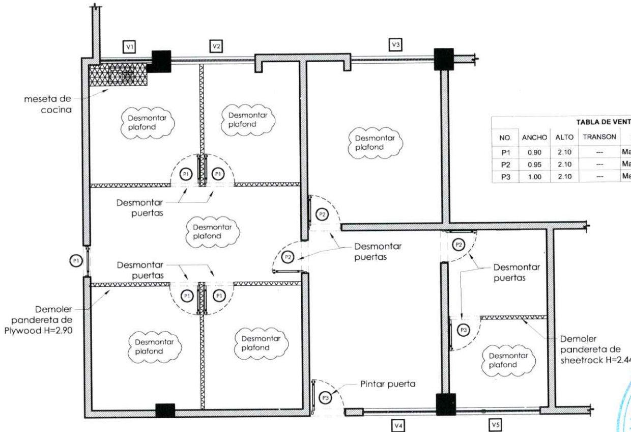
PLANTA: DE TRABAJO ESC: 1:100 1ER NIVEL
