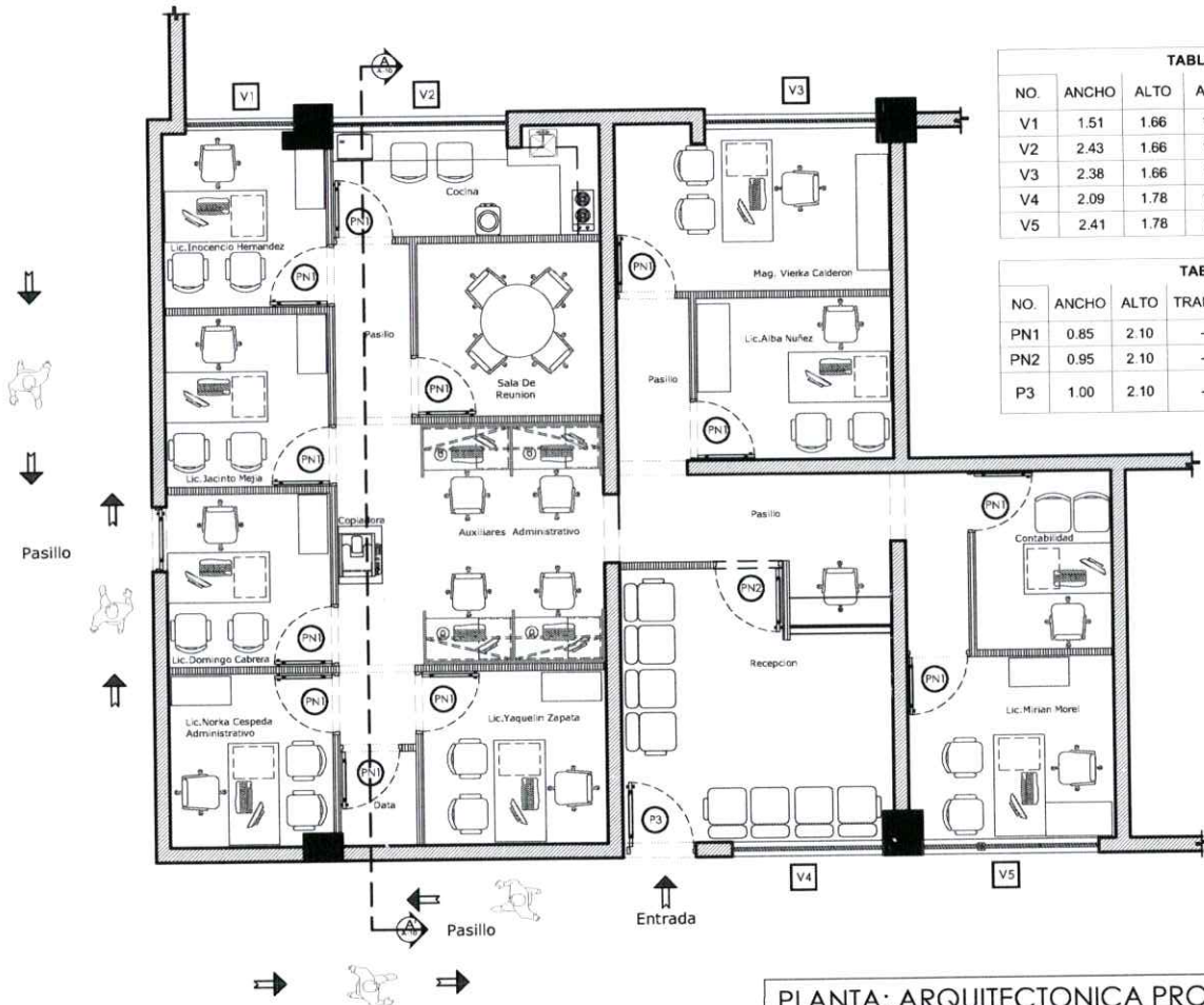
PLANTA: ARQUITECTONICA PROPUESTA ESC: 1:100 1ER NIVEL
