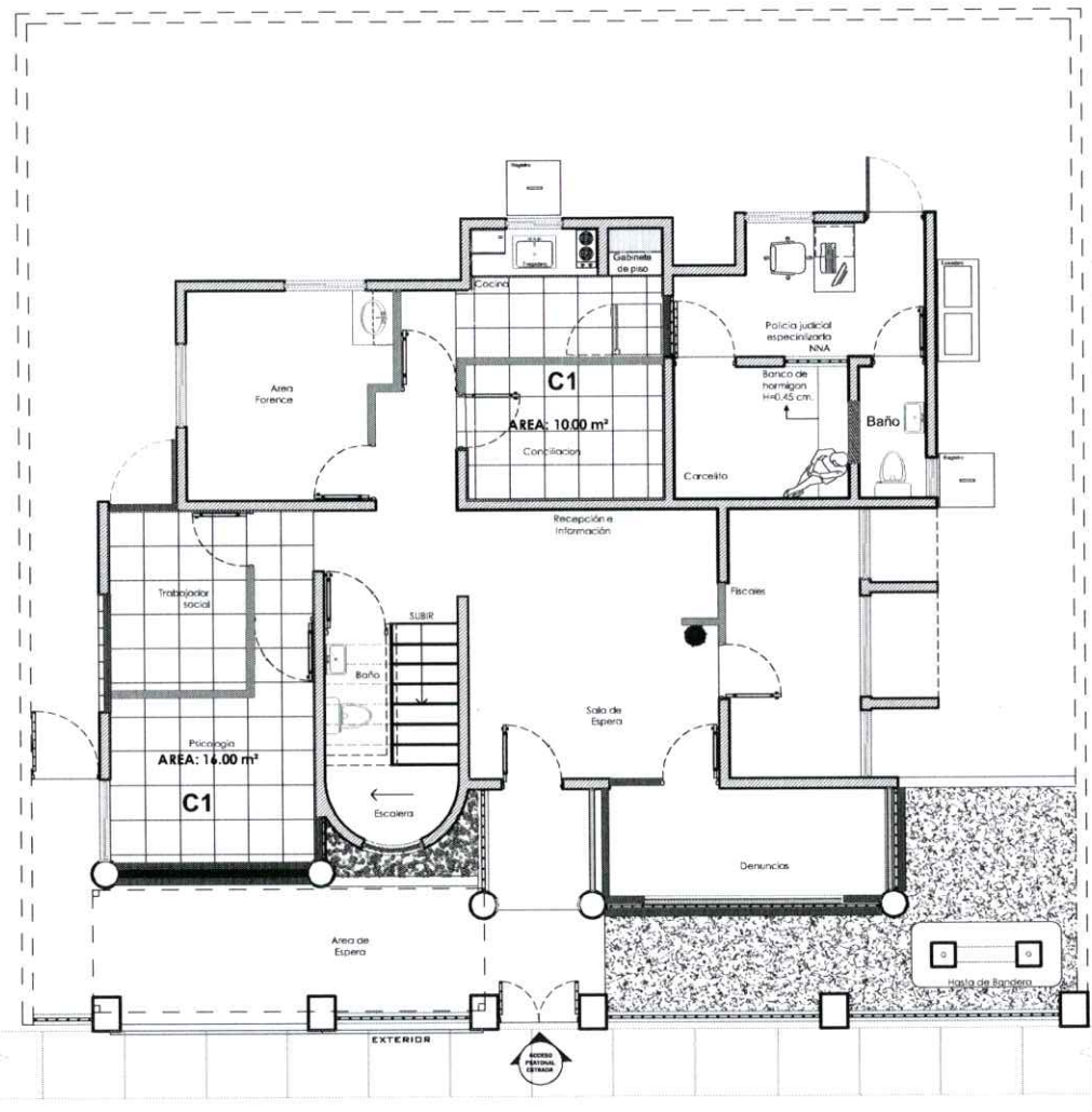
PLANTA: PLANO DE PISO 1ER. NIVEL. ESCALA: 1/75
