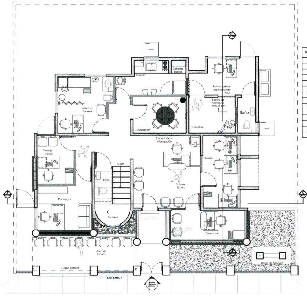
PLANTA: PLANO ARQUITECTONICO 3ER. NIVEL PROPUESTA ESCALA: 1/75
