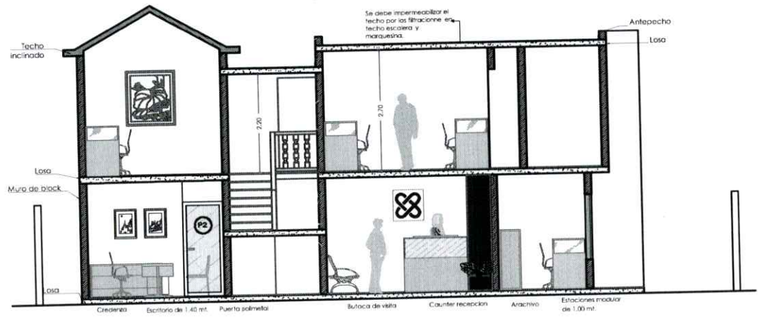
SECCIÓN: A-A ESCALA: 1/75
