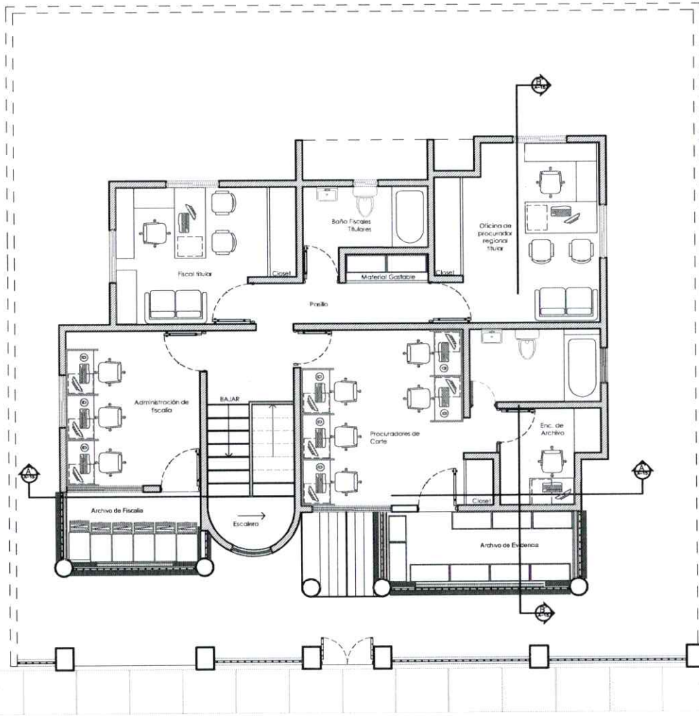
PLANTA: PLANO ARQUITECTONICO 200- NIVEL PROPUESTA ESCALA: 1/75
