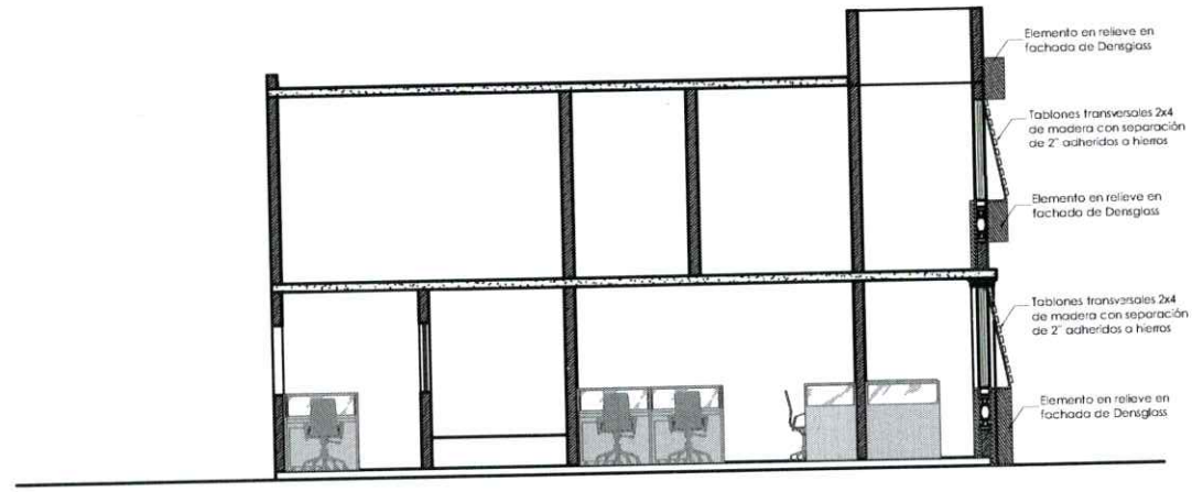
SECCIÓN: B-B ESCALA: 1/75
