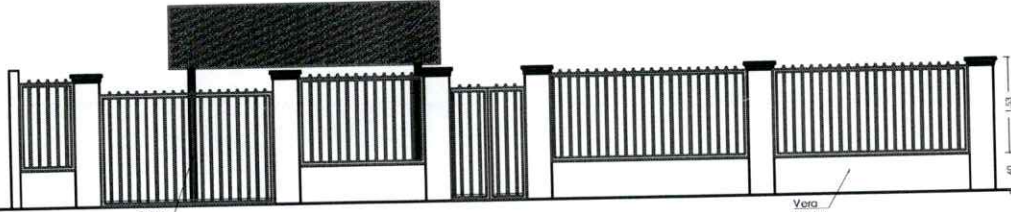
ELEVACIÓN: 1.FRONTAL DE VERJA (EXISTENTE) ESCALA: 1/75
